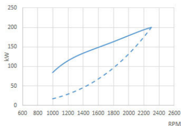
Effekt (ISO 3046/1)
